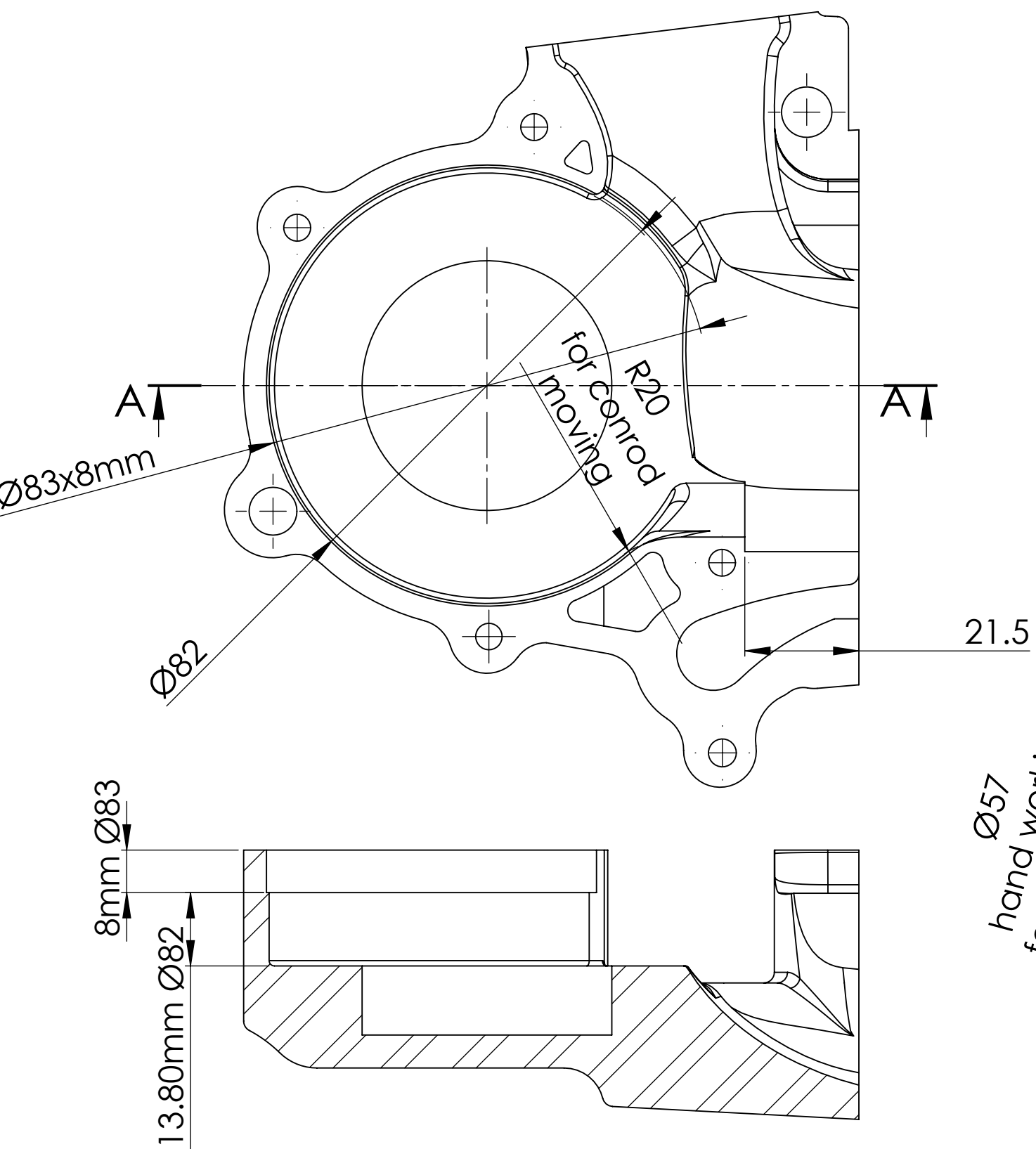
SEZIONE A-A
